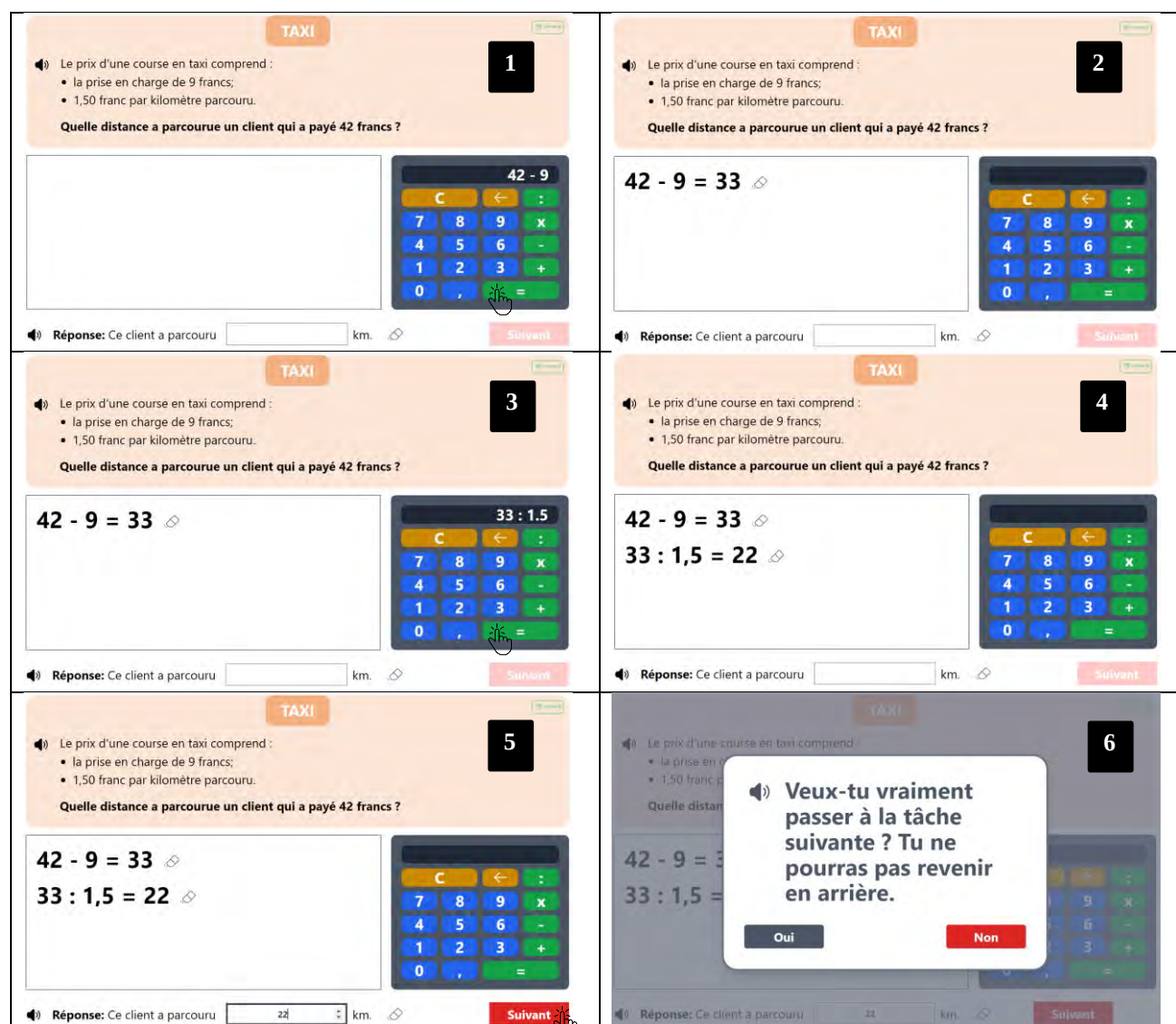
Fig. 2: Interaction du support numérique pour le problème Taxi
